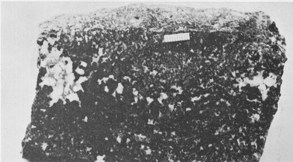
Sl. 2. Gabro. Jugovzhodno od Črne na Koroškem Abb. 2. Gabbro. Südöstlich Črna na Koroškem
