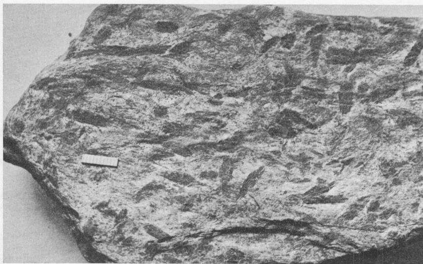
Sl. 2. Kontaktno metamorfoziran filit s porfiroblasti kordierita. Dolina Bistre pri Črni na Koroškem Abb. 2. Kontaktmetamorphosierter Phyllit mit Porphyroblasten von Cordierit. Bistra- Tal bei Črna na Koroškem
