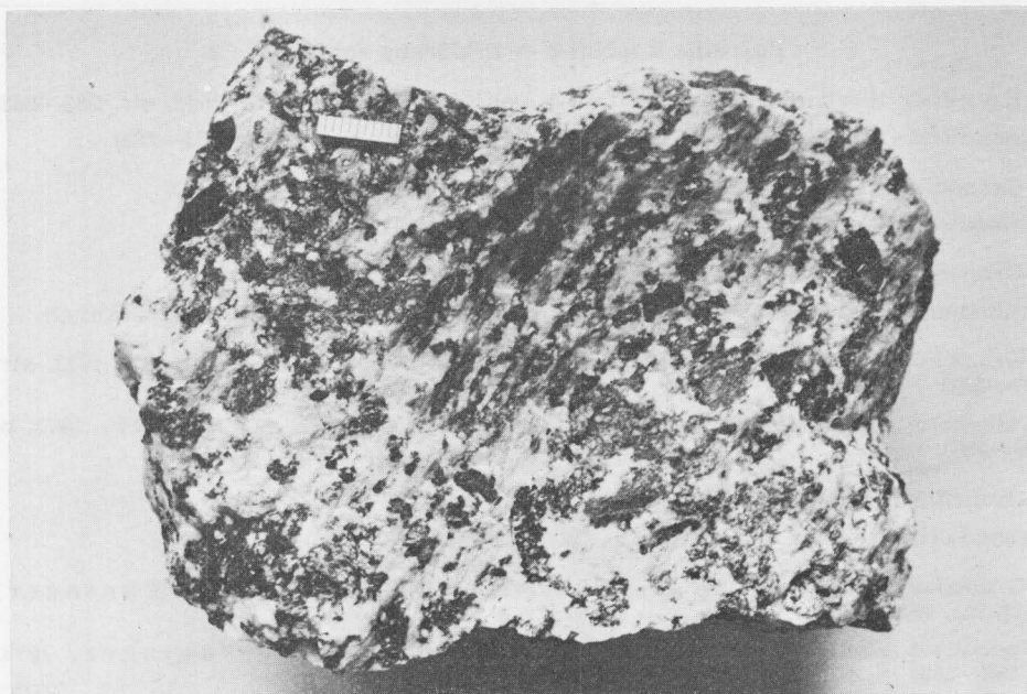
Sl. 1. Tonalit. Dolina Bistre pri Črni na Koroškem Abb. 1. Tonalit. Bistra-Tal bei Črna na Koroškem
