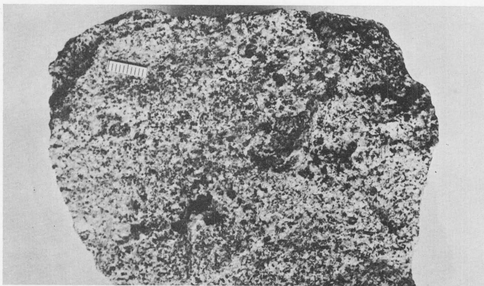
Sl. 2. Monzonitni diorit. Jugovzhodno od Črne na Koroškem Abb. 2. Monzodiorit. Südöstlich Črna na Koroškem
