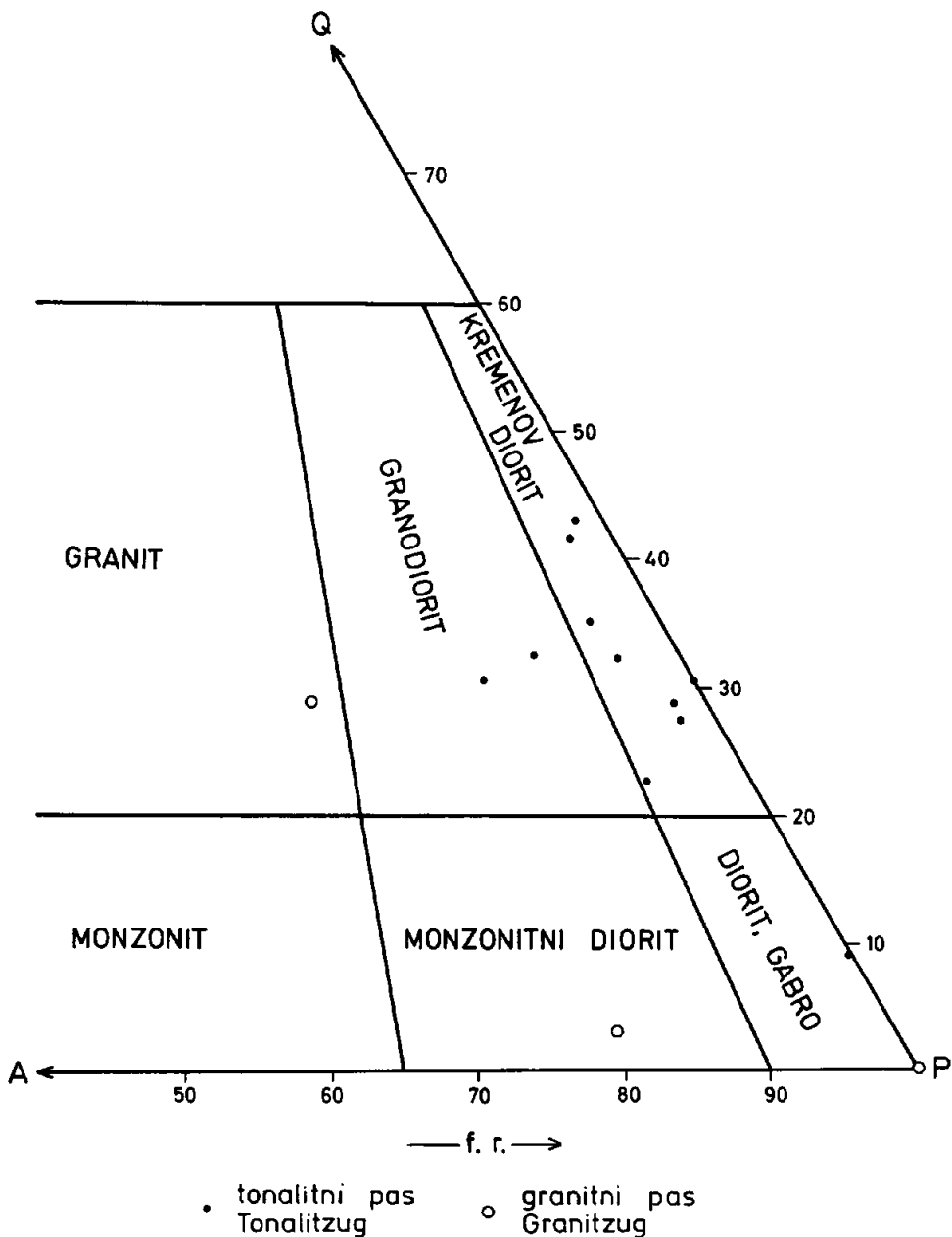
Sl. 2. Grafični prikaz vzorcev karavanške magmatske cone na diagramu Q-A-P (Streckeisen, 1967)
