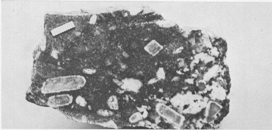
Sl. 1. Porfiroidni monzonitni diorit. Jugovzhodno od Črne na Koroškem Abb. 1. Porphyroider Monzodiorit. Südöstlich Črna na Koroškem
