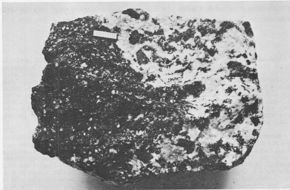
Sl. 2. Melanokratni vključek v tonalitu. Dolina Bistre pri Črni na Koroškem Abb. 2. Melanokrater Einschluß im Tonalit. Bistra-Tal bei Črna na Koroškem
