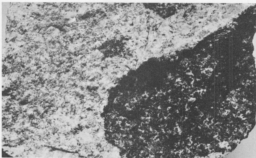
Sl. 1. Magmatska breča — odlomki gabra v granitu (naravna velikost). Topla Abb. 1. Magmatische Breccie — Bruchstücke von Gabbro im Granit (natürliche Größe). Topla
